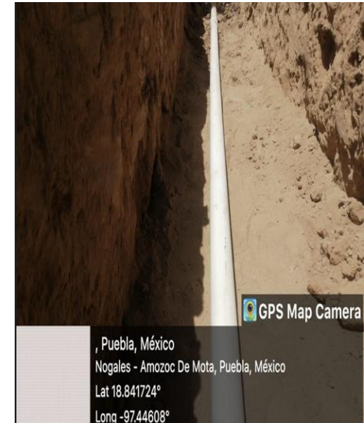
INSTALACIÓN DE TUBERÍA DE 2” DE DIÁMETRO EN RED DE DISTRIBUCIÓN
